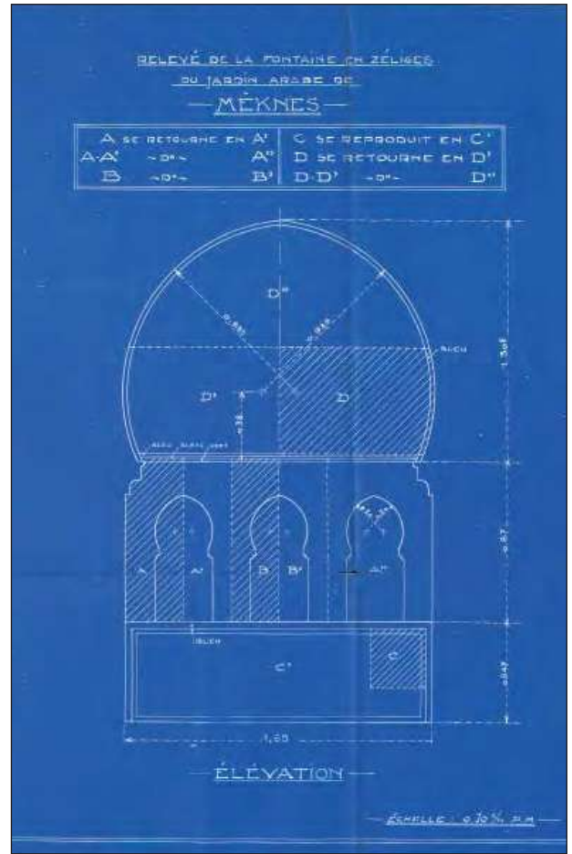
مسح معماري لسقاية بالحديقة العمومية بمكناس.
